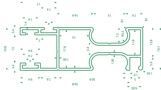
GC-15328 Altınsin Sürme Kanat Ağırlık 0,737 Kg
